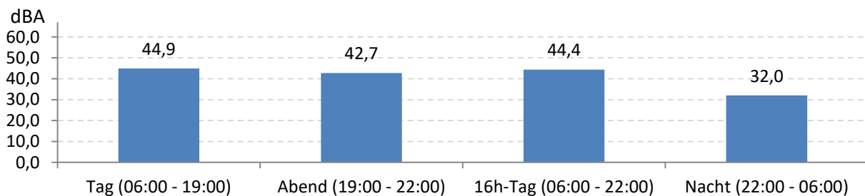
Abb. 8: LEQ bei Pistenbetriebsrichtung "Windstille" 186 Stunden im Messzeitraum
