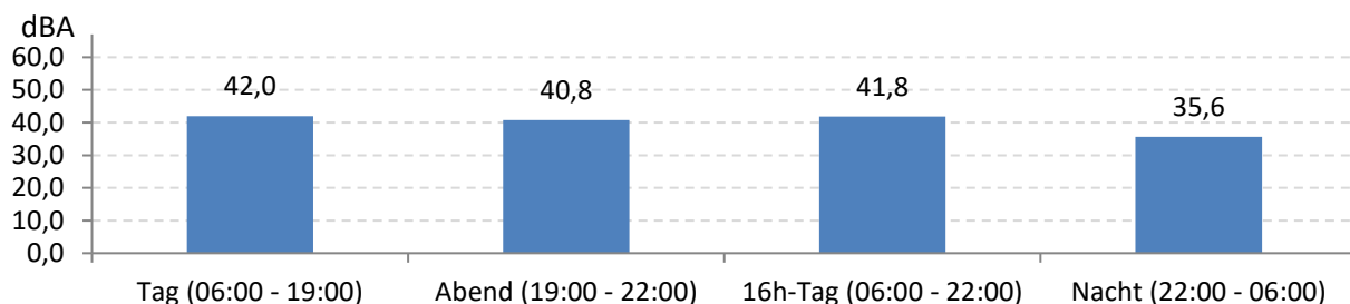
Abb. 9: LEQ bei Pistenbetriebsrichtung "östliche Winde" 351 Stunden im Messzeitraum
